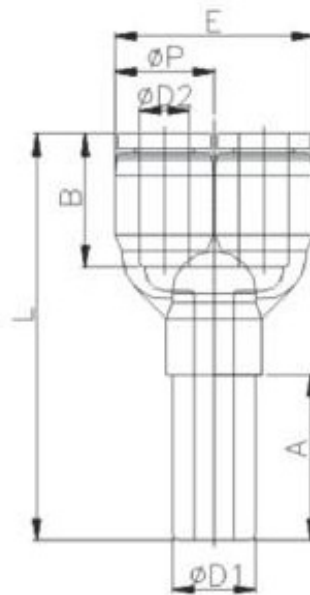
Diagram - Plug-In Y (PYJ)
